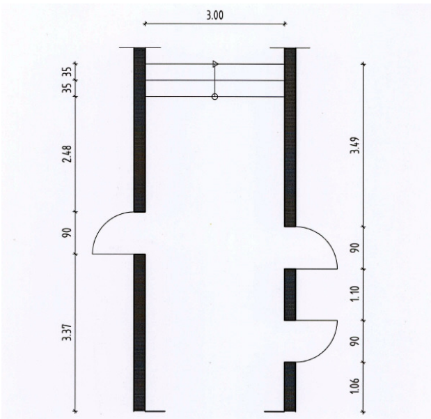
Grundriss Ausstellungsraum
